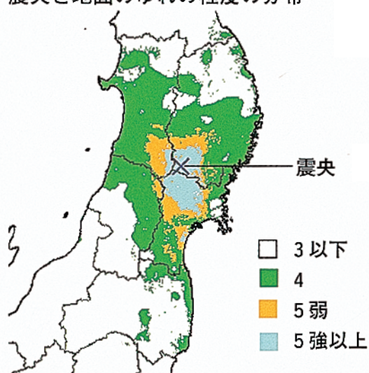
図1 震央と地面のゆれの程度の分布
