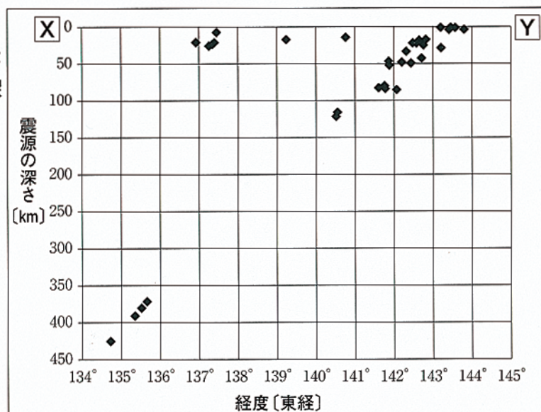
図3 X-Y付近に起きた 主な地震の震源の深 さの分布
