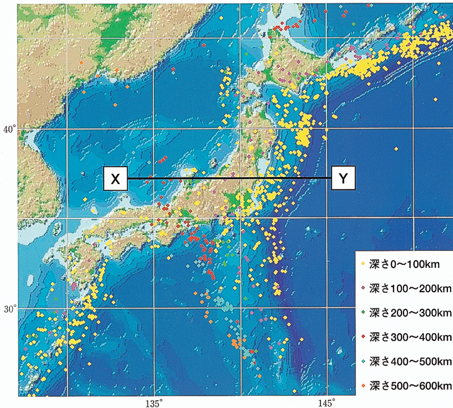
図2 日本付近の地震の震源の分布 (1984年～1999年)
